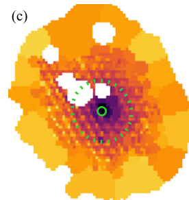
\log \Sigma_{\star} [M_{\odot} \text{pc}^{-2}]
