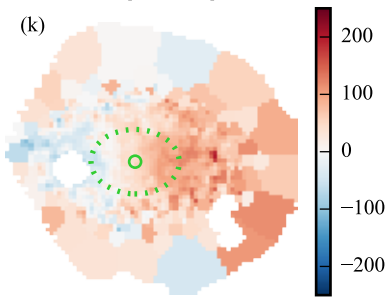
v_{\star} [\text{kms}^{-1}]
