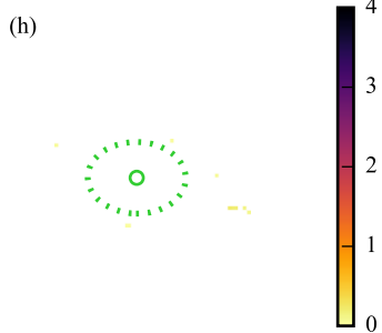
v_{\star} [\text{kms}^{-1}]
