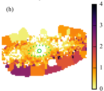
v_{\star} [\text{kms}^{-1}]
