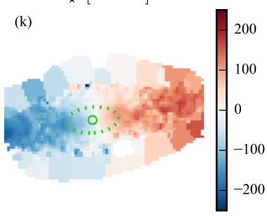
v_{\star} [\text{kms}^{-1}]
