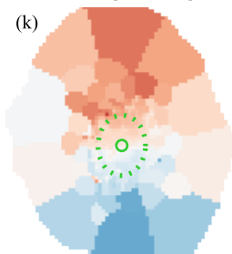
v_{\star} [\text{km s}^{-1}]
