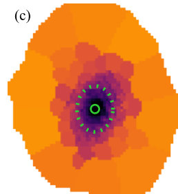
\log \Sigma_{\star} [M_{\odot} \text{pc}^{-2}]
