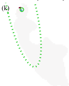
v_{\star} [ \text{km s}^{-1} ]
