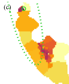
\log \Sigma_{\star} [ M_{\odot} \text{pc}^{-2} ]
