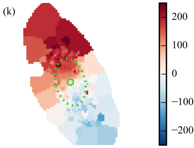
v_{\star} [\text{km s}^{-1}]
