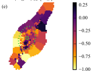
b^{\text{loc}}
