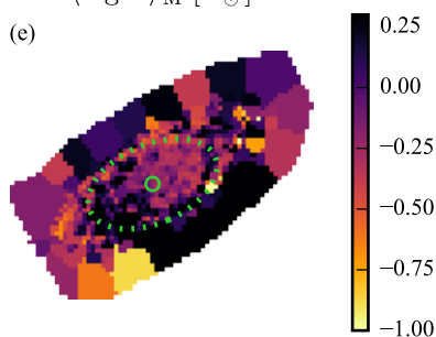
b^{\text{loc}}
