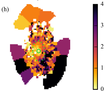
b^{\text{loc}}
