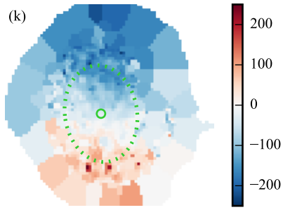
v_{\star} [\text{kms}^{-1}]
