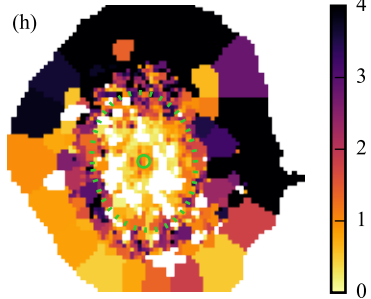
v_{\star} [\text{kms}^{-1}]
