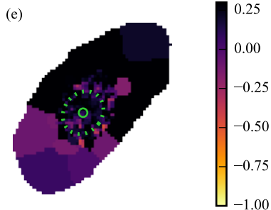
b^{\text{loc}}
