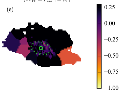
b^{\text{loc}}
