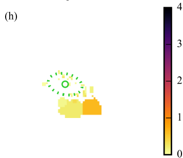
v_{\star} [\text{km s}^{-1}]
