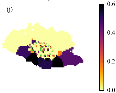
\tau_{\text{V}}
