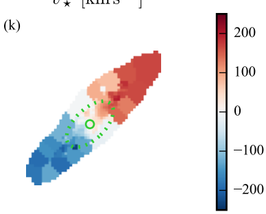
v_{\star} [\text{km s}^{-1}]
