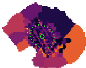
b^{\text{loc}}
