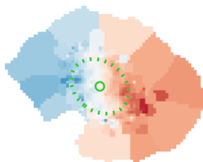
v_{\star} [ \text{km s}^{-1} ]
