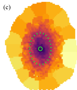
\log \Sigma_{\star} [\text{M}_{\odot} \text{pc}^{-2}]
