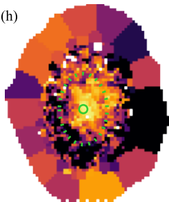
v_{\star} [\text{km s}^{-1}]
